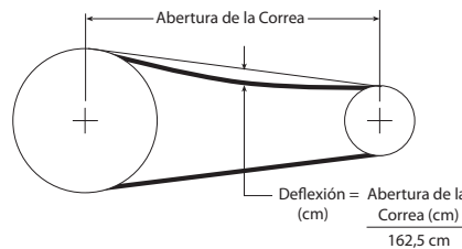
Figura 7 — Tensión de la Correa
