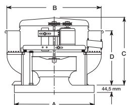
Figura 1 — Dimensiones
